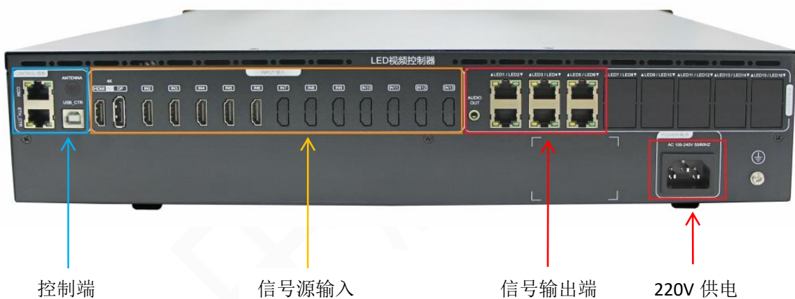
后面板
